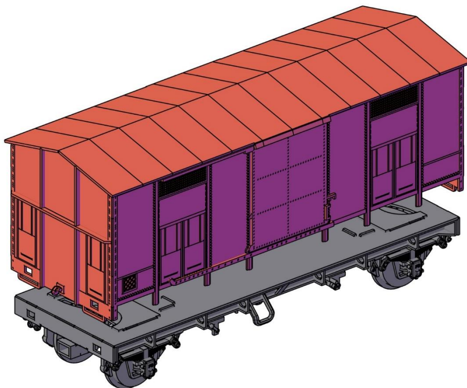
Passo 64 – Inserire la cassa sopra al telaio
