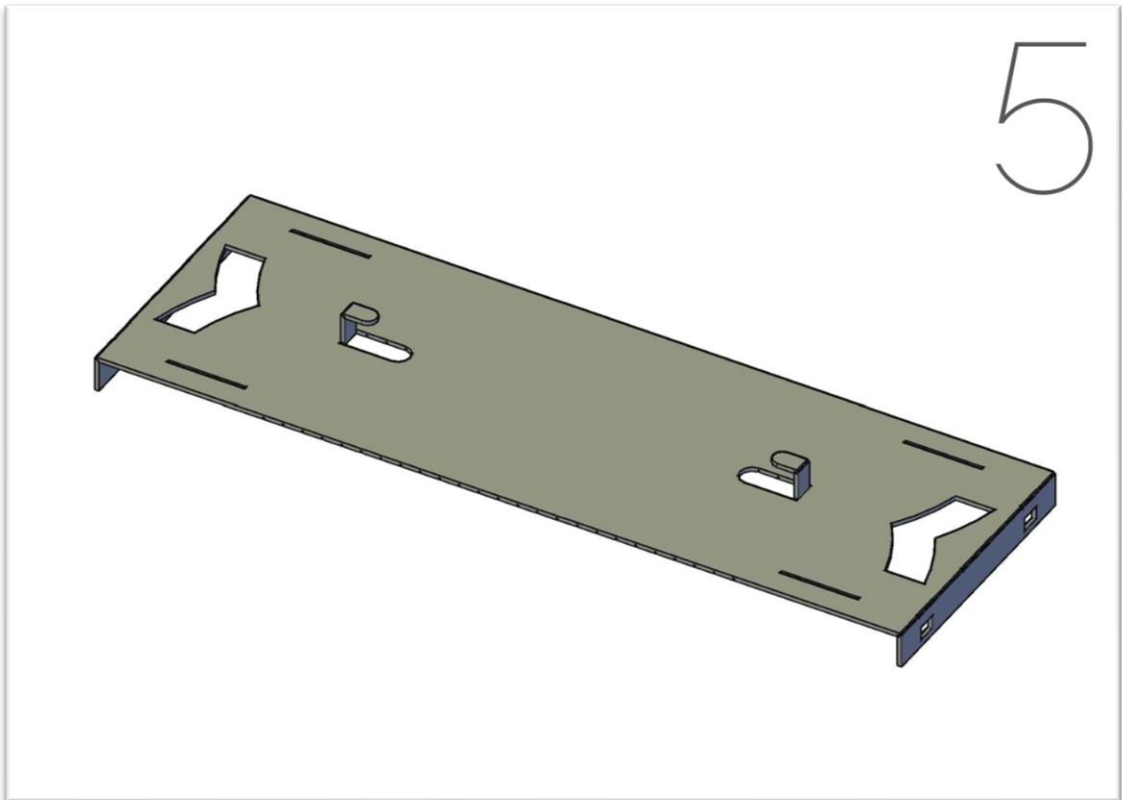
5. Piegare i fermi per la molla del portagancio
