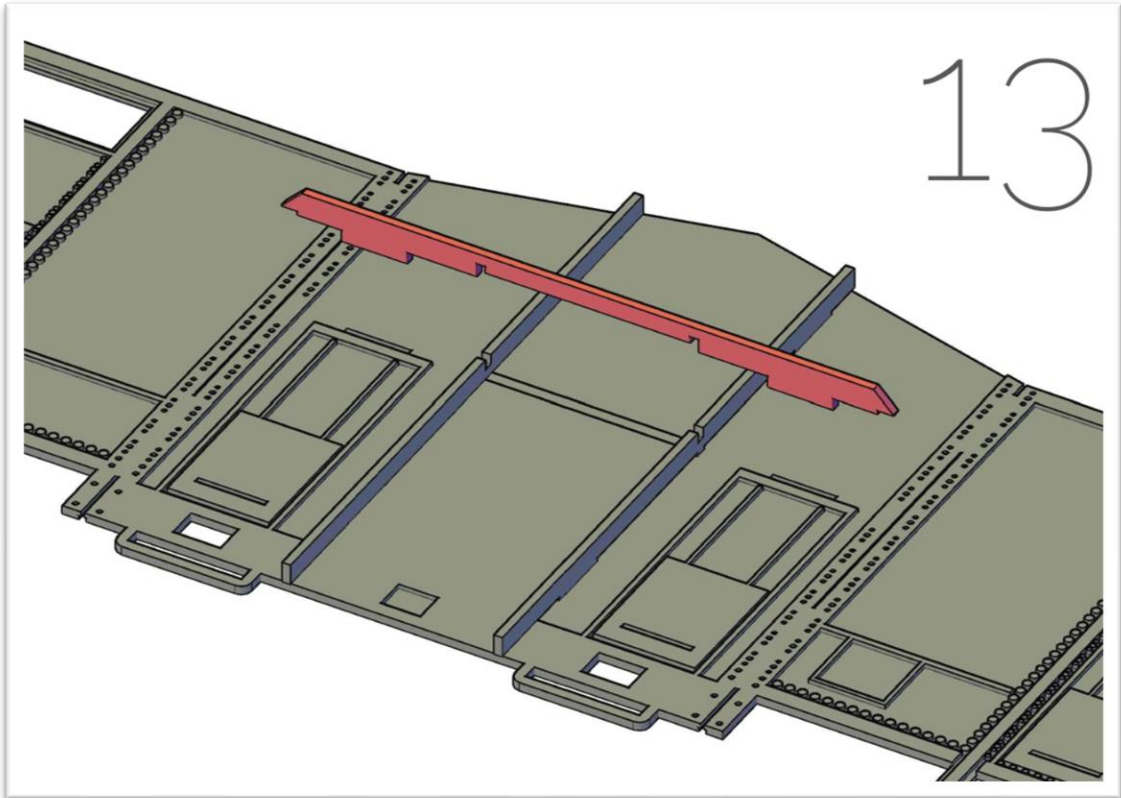
13: Inserire i rinforzi orizzontali e ripetere per entrambe le testate
