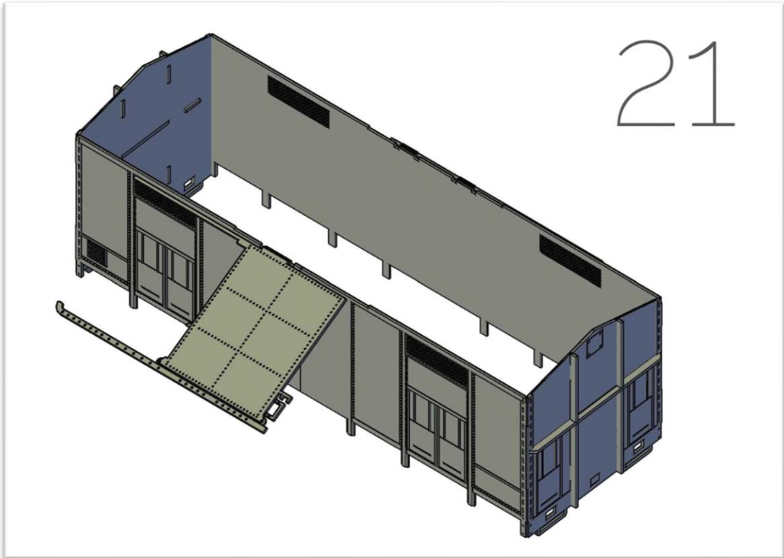
21: Piegare verso il basso i portelloni
