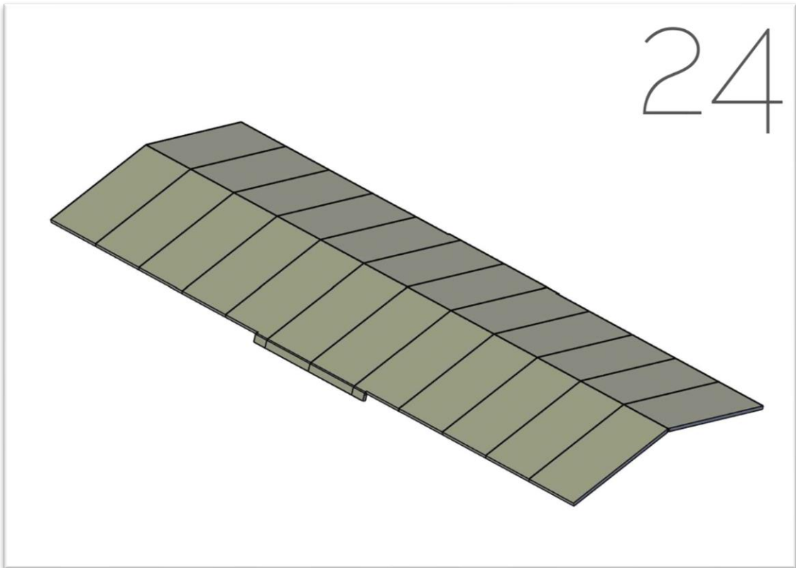
24: Piegare verso il basso le coperture dei portelloni
