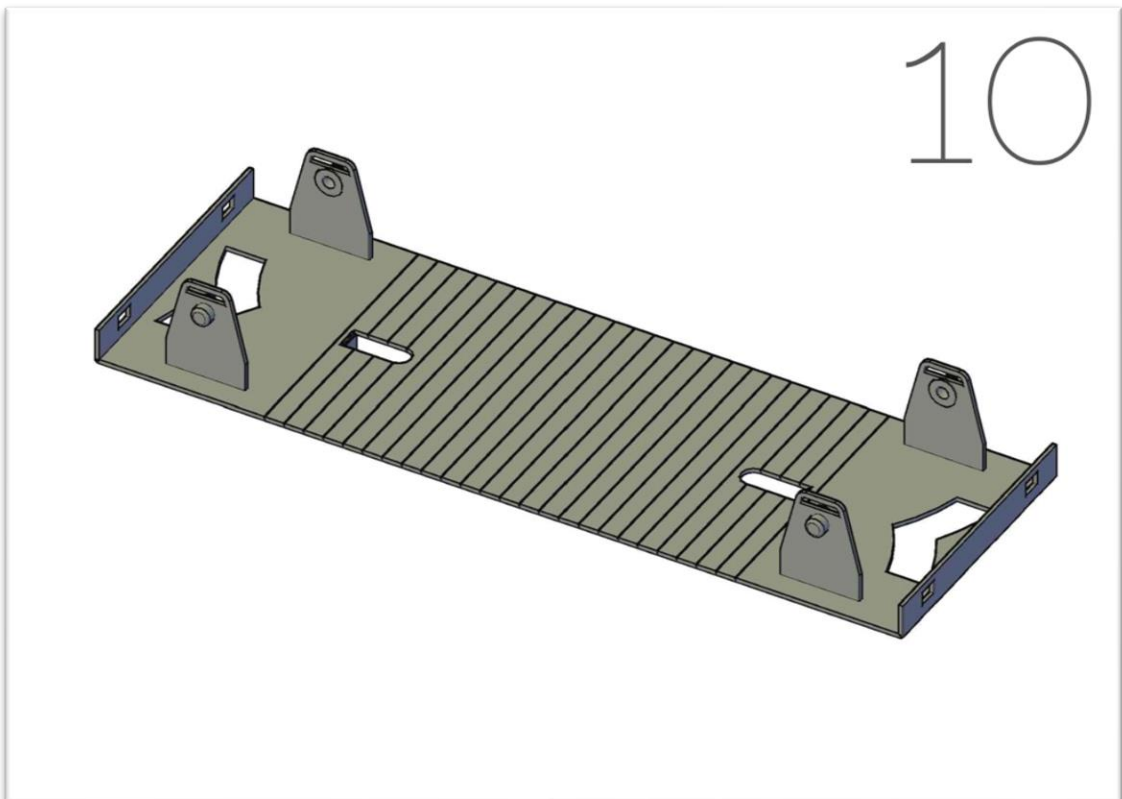
9-10. Inserire e fissare le boccole coniche
