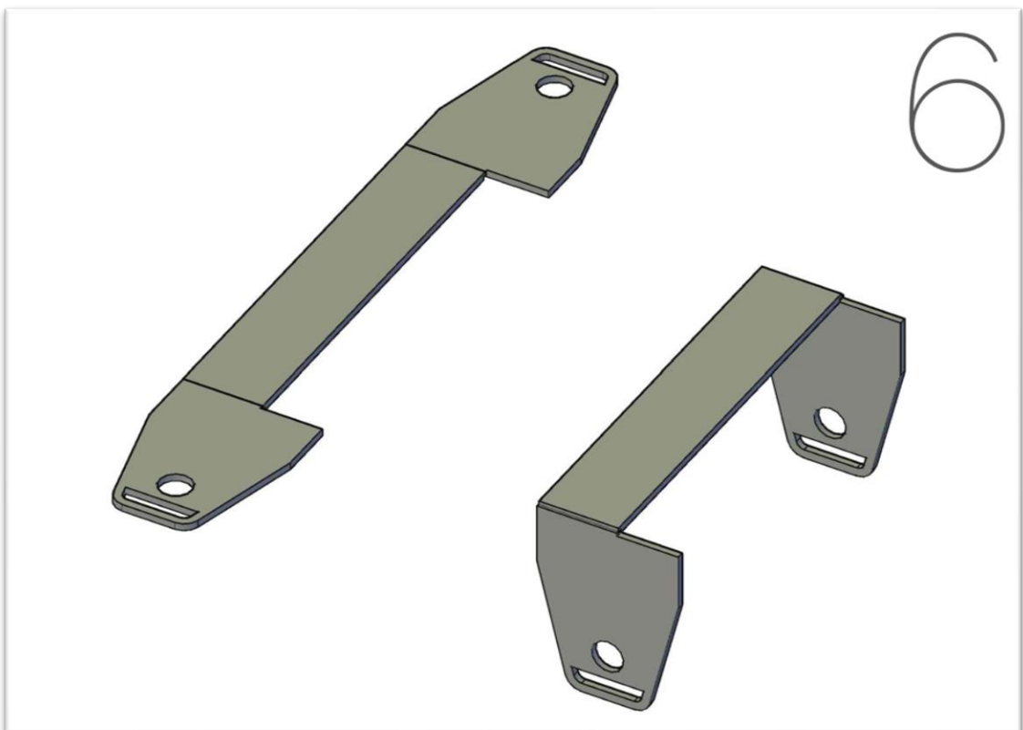
6. Piegare a "U" i supporti degli assali (ripetere 2 volte)
