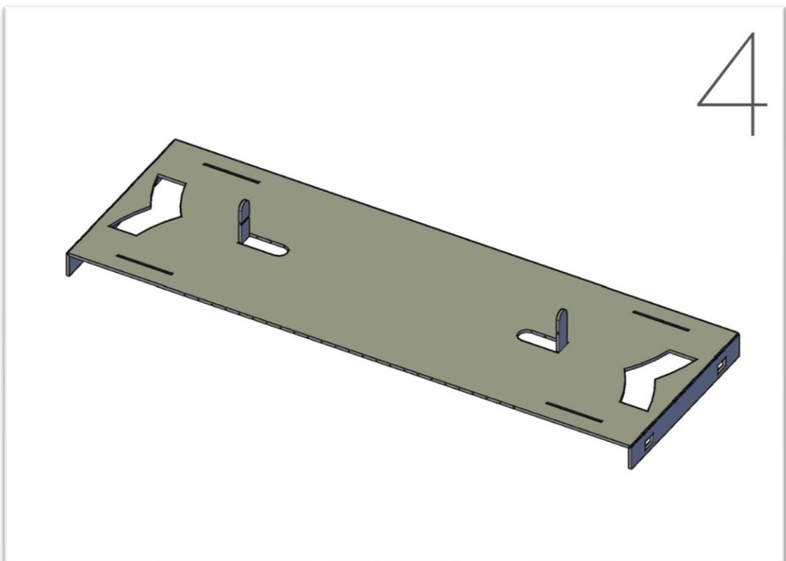
4. Piegare i fermi per la molla del portagancio
